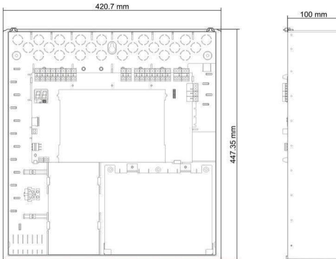
Obrázek 24: Osmizónová skříň bez krytu
