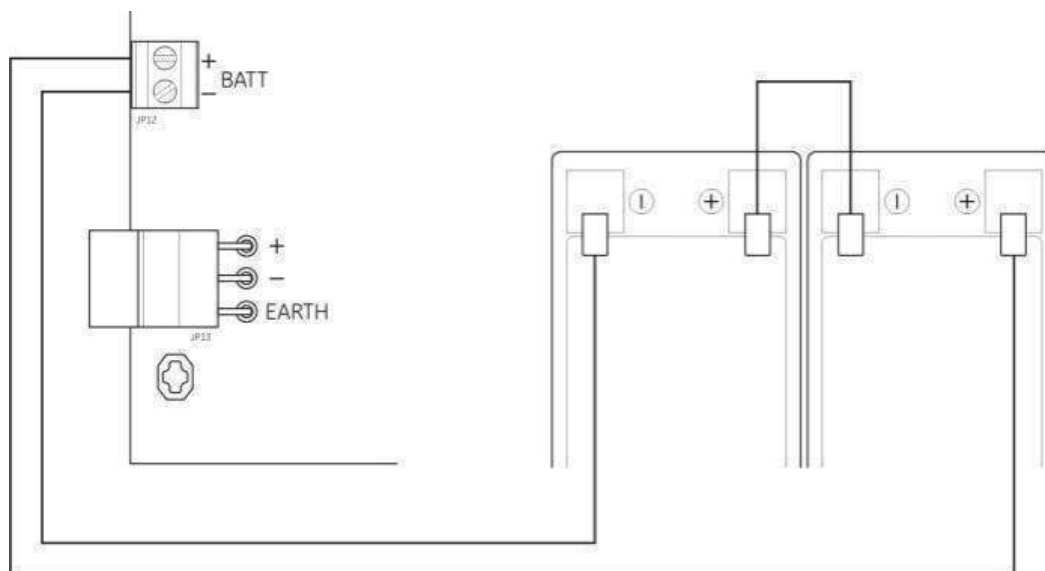
Obrázek 12: Připojení baterií
